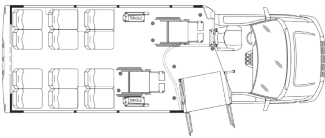
24', 12+4 Passenger, 2 w/c
